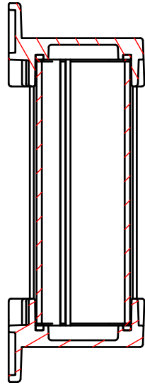
B-B (1:2)
